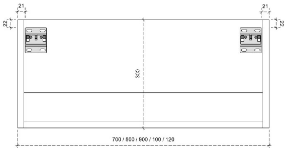
DETAILS onderkast met 1 lade DIEPTE 45
