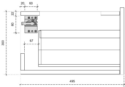
DETAILS onderkast met 1 lade DIEPTE 50
