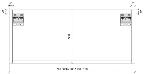
DETAILS onderkast met 1 lade DIEPTE 50
