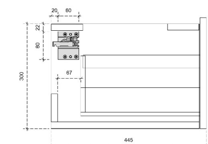
DETAILS onderkast met 1 lade DIEPTE 45
